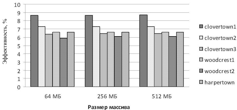
Рис. 4. Эффективность задачи для процессоров линейки Xeon
