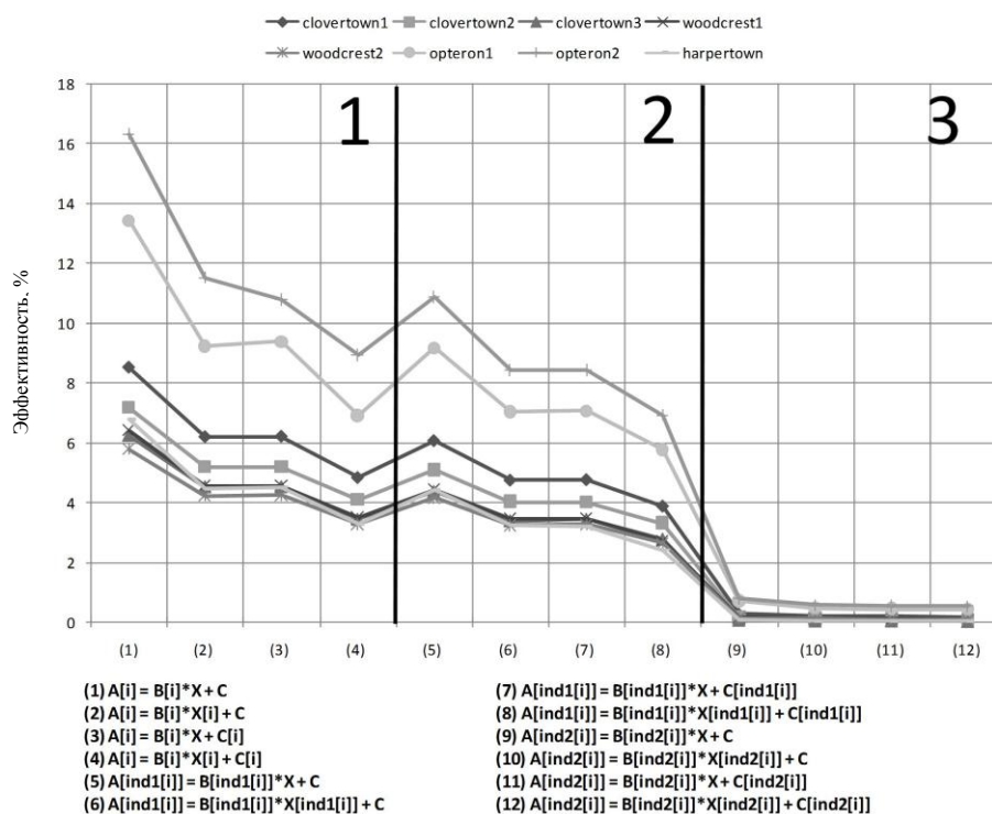
Рис. 5. Влияние степени локальности данных на эффективность реализации «триады»
