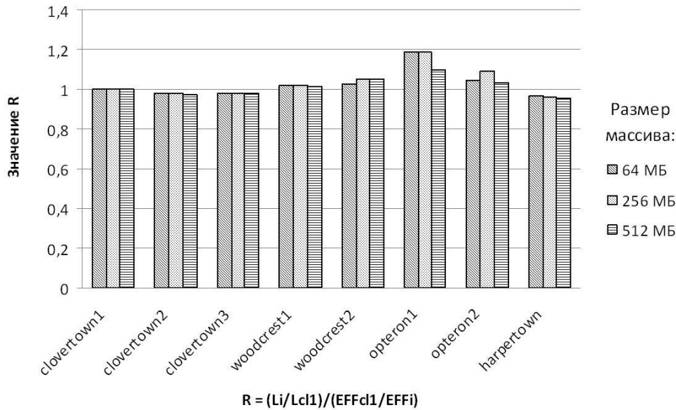
Рис. 3. Влияние характеристики L на эффективность реализации структуры «триада»
