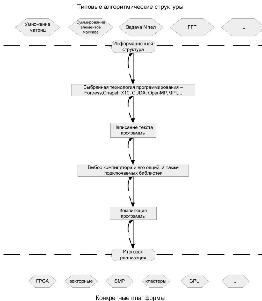
Рис. 1. Общая схема отображения типовых алгоритмических структур на вычислительные системы
