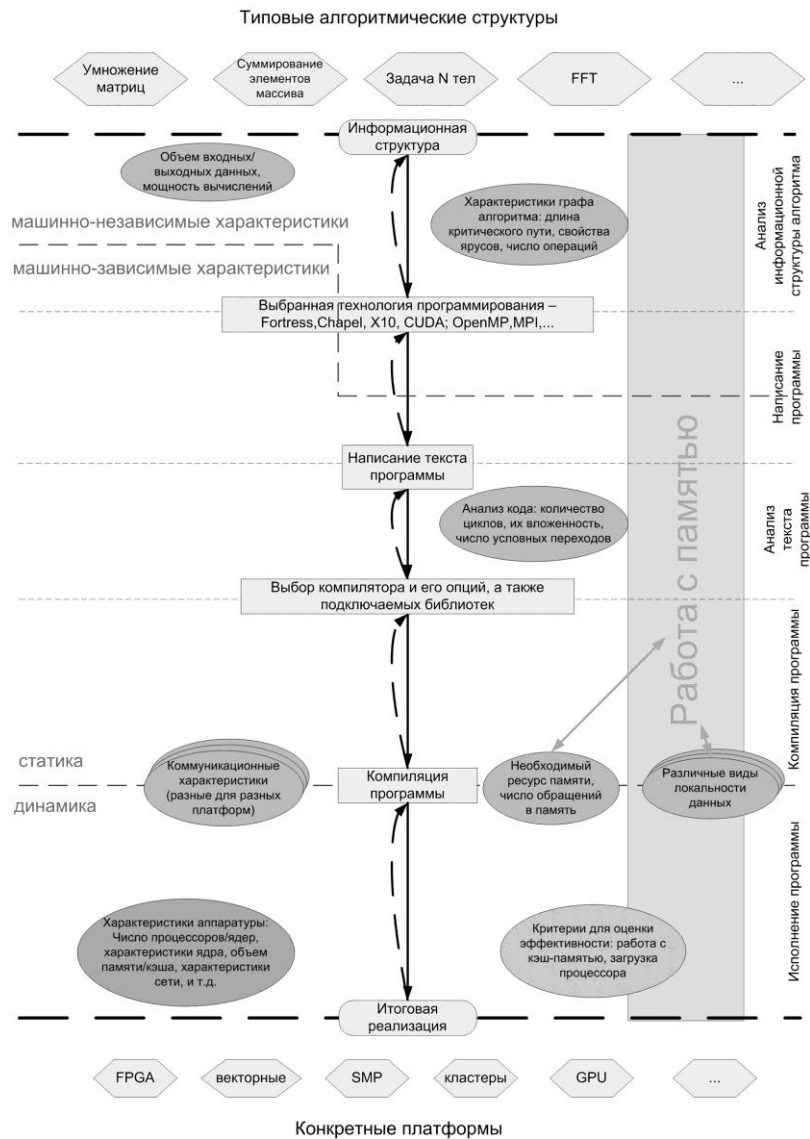
Рис. 2. Основные характеристики различных этапов отображения типовых алгоритмических структур
